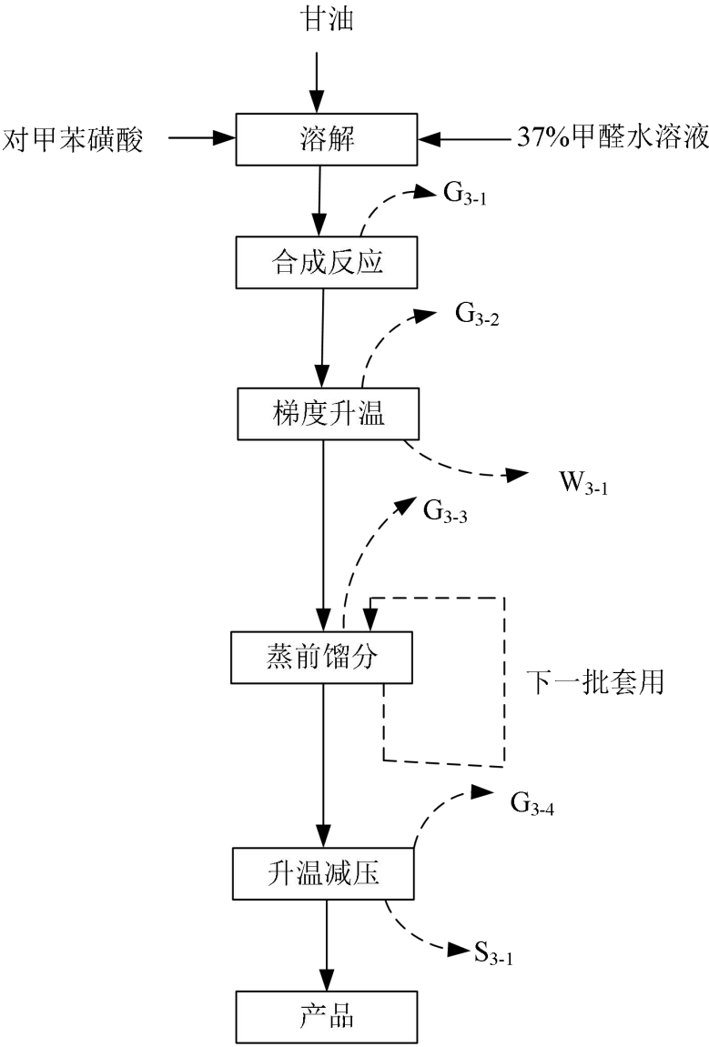
甘油缩甲醛制备生产工艺流程及产污节点示意图
