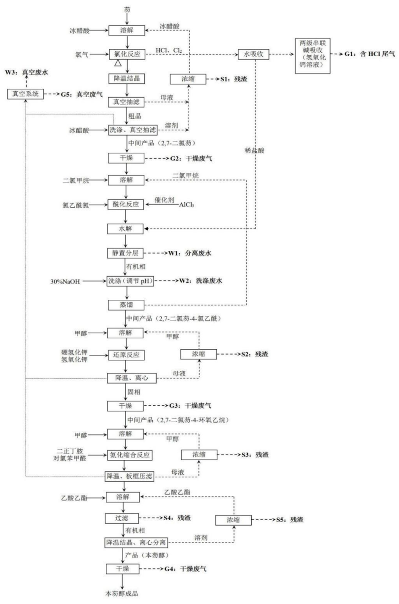
图 1 本茆醇生产工艺流程图
