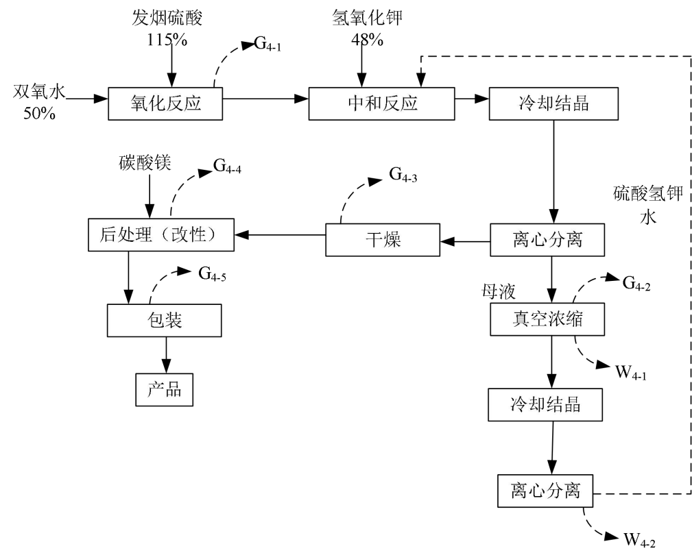
过一硫酸氢钾复合盐制备生产工艺流程及产污节点示意图
