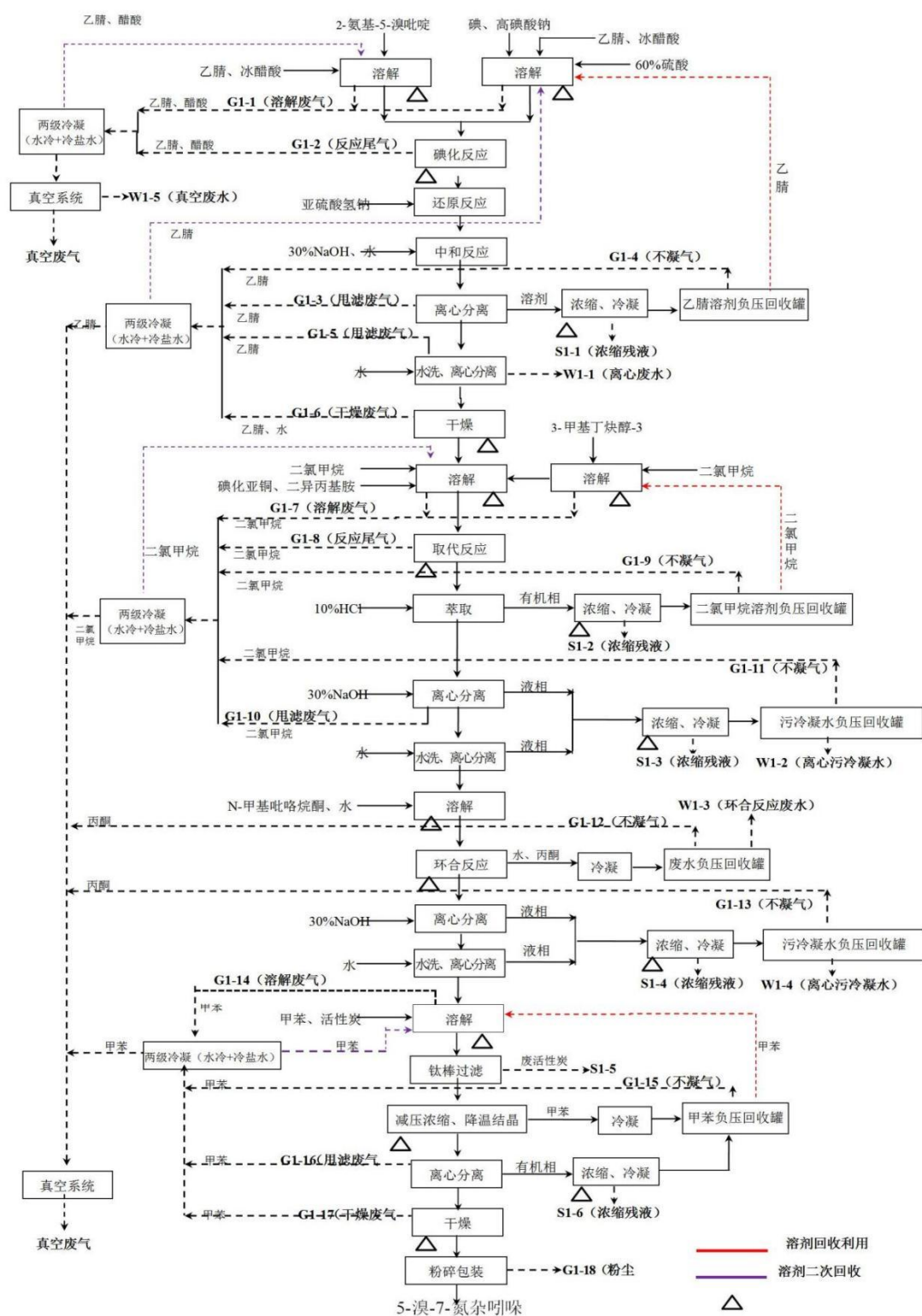
5-溴-7-氮杂吡啶生产工艺流程及产污环节图见下图。
